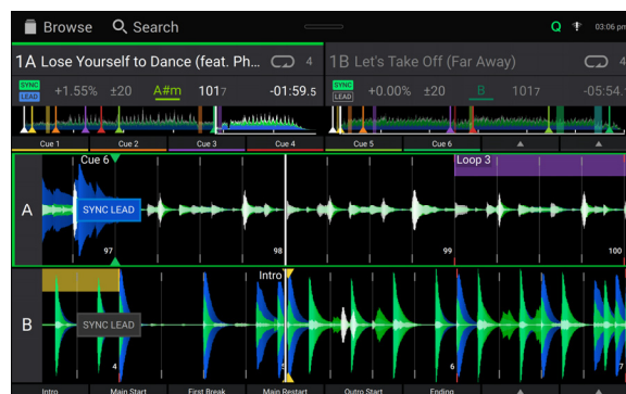
Visualizzazione delle onde a strato doppio
